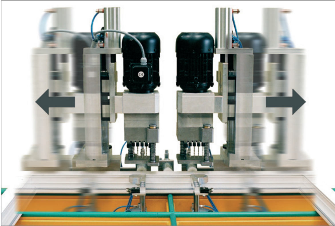
Bohrereinheit mit feststehendem oder automatisch drehbarem Sechsspindel-Bohrkopf und federbelasteter Bohrbrille
