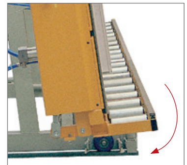
Abbildung mit pneumatisch abklappbarer Rollenbahn
